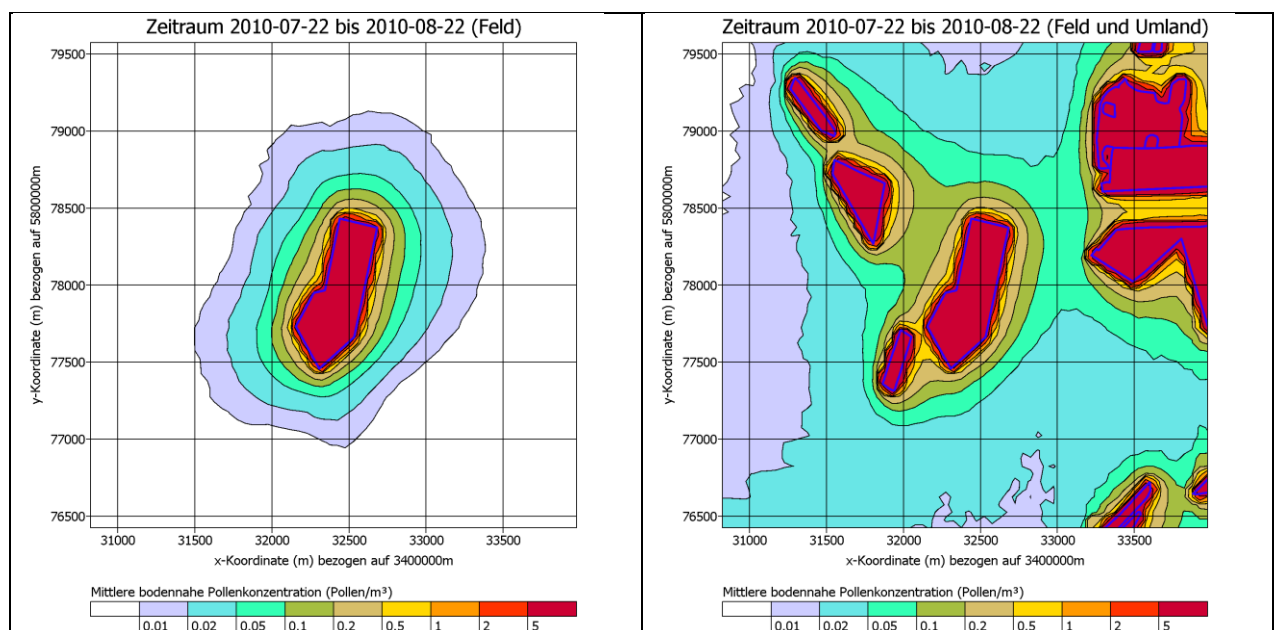
Abb. 64: Modellerte bodennahe Konzentrationsverteilung der Pollen (Mittelwert über den Zeitraum 22.07.2010 bis 22.08.2010). Links: Nur Beiträge vom Versuchsfeld. Rechts: Beiträge von Versuchsfeld und Umlandfeldern. (Grafiken: Janicke)
