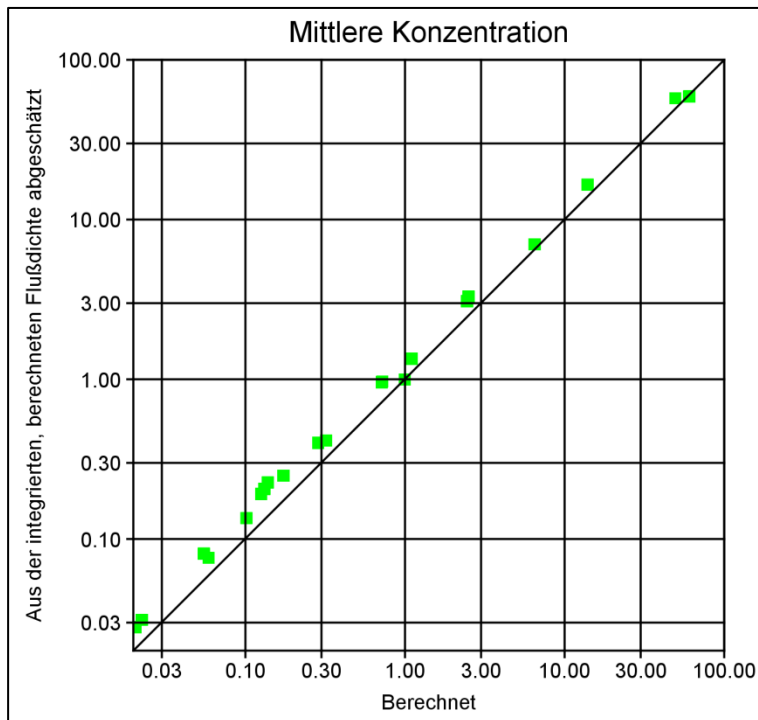
Abb. 63: Streudiagramm von berechnetem Konzentrationsmittel und dem aus der integrierten, berechneten Flußdichte abgeschätzten Konzentrationsmittel. (Grafik: Janicke)
